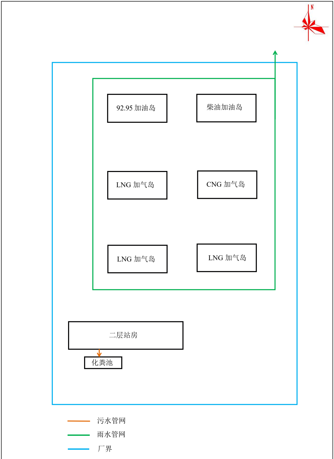
附图 3 厂区平面布置及雨污管网图
